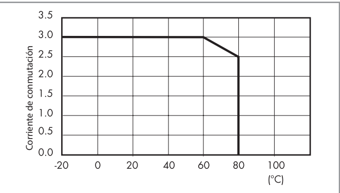
L 41 - Corriente de conmutación en función de la temperatura ambiente - SSR - Salida 3 A AC
