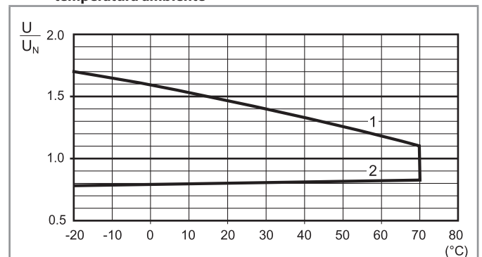
R 66 - Campo de funcionamiento de la bobina AC en función de la temperatura ambiente
